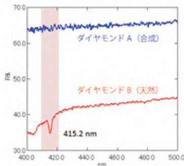
ダイヤモンドの紫外可視反射スペクトル測定 青:合成ダイヤモンド 赤:天然ダイヤモンド
